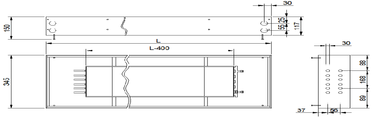
DT DK12-DK 22-DK32 MODELİ DÖŞEME KONVEKTÖRÜ SEÇİM TABLOSU
